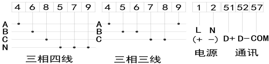
交直流辅助电源或带通讯的 09 外形电压表接线图
