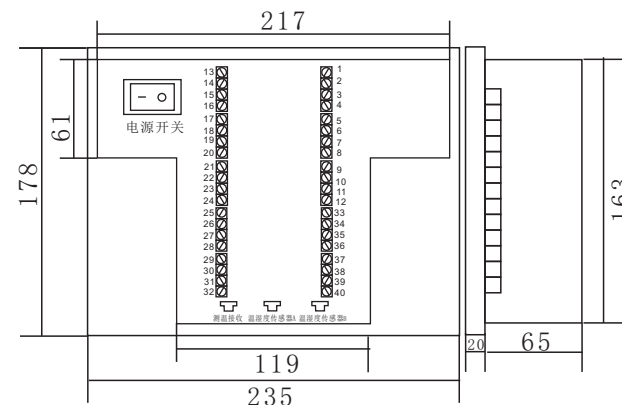
外形尺寸: 235×178×85
