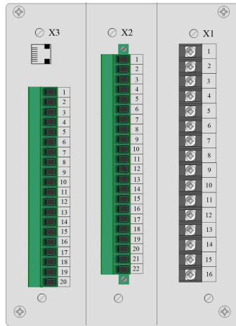
背视图
