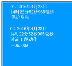
图 5.5-6 事故记录画面图
