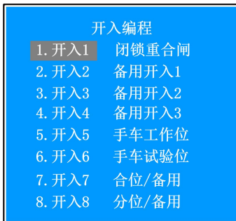
图 5.4 -16 遥信时间设置画面图
